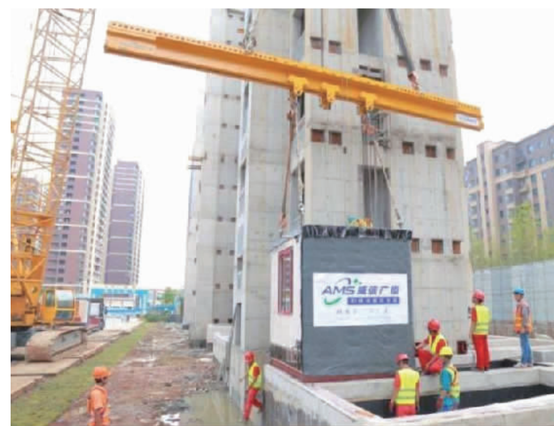
图为施工现场。顾宗侠 摄
